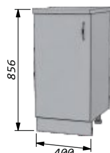
Стол 40 без ящика правый/ левый Ширина - 400мм Высота - 856мм Глубина: по столешнице - 600мм по корпусу - 460мм
