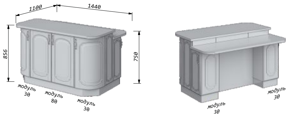
Кухонный остров тип 4 - обеденный с радиусным фасадом (только МДФ)
