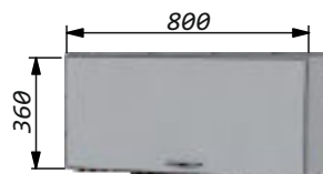
Шкаф глухой под вытяжку 80 («Хлебница») открывается вверх. Ширина -800мм Высота -360мм Глубина-270мм
