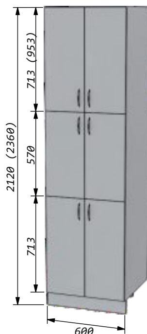
Пенал 60 шесть дверей Ширина -600мм Высота -2120мм Глубина-561мм
