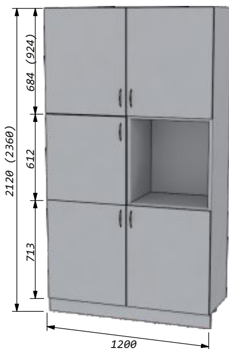
Пенал-встройка 120 пять дверей правый/левый Ширина - 1200мм Высота - 2120мм Глубина - 561мм
