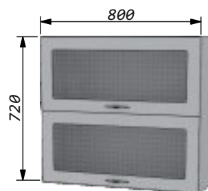
Шкаф-витрина 80 х2 с 2 стеклами открывание вверх Ширина - 800мм Высота - 720мм Глубина - 270мм
