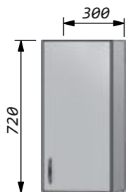
Шкаф-скос 30 с фасадом (петли 30 градусов) Ширина -300мм Высота -720мм Глубина-270мм
