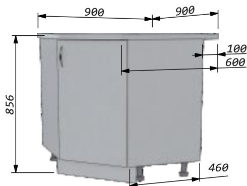
Стол угловой скошенный 90x90 правый/левый Размер: по столешнице - 900x900мм по корпусу - 800x800мм Глубина: - по боковому срезу столешницы - 600мм - по боковине корпуса - 460мм Ширина фасада: - 451мм Длина цоколя - 497мм
