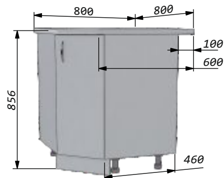
Стол угловой скошенный 80х80 правый/левый Размер: по столешнице - 800х800мм по корпусу - 700х700мм Глубина: - по боковому срезу столешницы - 600мм - по боковине корпуса - 460мм Ширина фасада - 310мм Длина цоколя - 355мм
