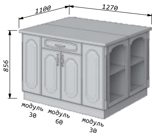
Кухонный остров тип 6 (одноуровневый с торцевыми рамками)
