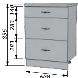
Стол 60 с тремя ящиками Ширина - 600мм Высота - 856мм Глубина: по столешнице - 600мм по корпусу - 460мм
