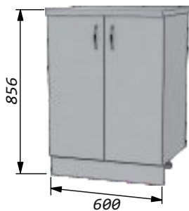
№00 Стол 60 без ящика. Ширина - 600мм Высота - 856мм Глубина: по столешнице - 600мм по корпусу - 460мм
