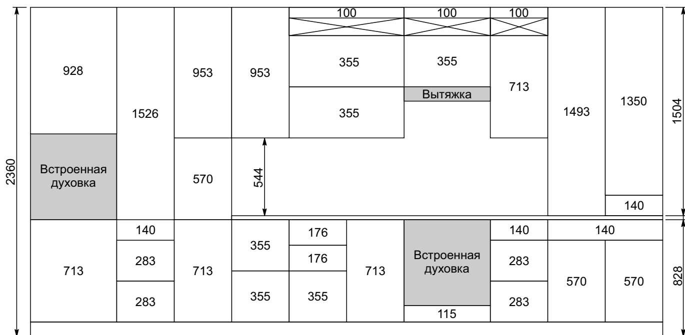
Типовые высоты фасадов (верх 960, столешница 28 мм)
