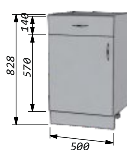
№011 правый/левый Стол-мойка 50 с фальш ящиком, левый. Ширина - 500мм Высота - 856мм Глубина: по корпусу - 460мм
