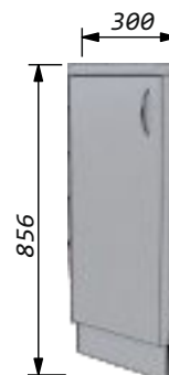
Шкаф-скос 30 с фасадом (петли 45 градусов) Ширина -300мм Высота -856мм Глубина: по столешнице-600мм по корпусу -561мм Применяется в сочетании с шкафом-скосом 30 граненым или скругленным
