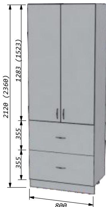
Пенал 80, два ящика + две двери Ширина - 800мм Высота - 2120мм Глубина - 561мм
