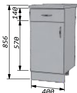
Стол 40 с одним ящиком правый/левый Ширина - 400мм Высота - 856мм Глубина: по столешнице - 600мм по корпусу - 460мм
