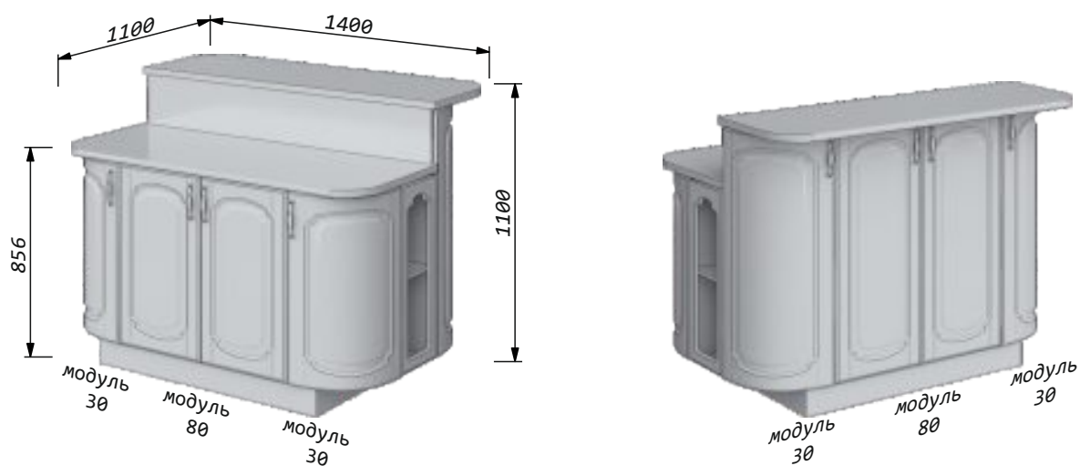
Кухонный остров тип 4 - обеденный с радиусным фасадом (только МДФ)
