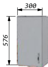
Шкаф 30 правый/левый Ширина - 300мм Высота - 576мм Глубина - 270мм
