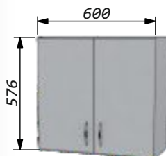
Шкаф 60. Ширина - 600мм Высота - 576мм Глубина - 270мм
