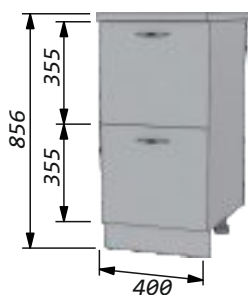
Стол 40 с двумя ящиками.
