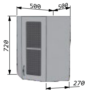
Шкаф-витрина угловой 50x50 правый/левый Ширина - 500x500мм Высота - 720мм Глубина - 270мм
