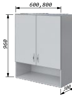
Шкаф х2 глухой 60/80 открывание вверх Ширина - 600/800мм Высота - 960мм Глубина - 300мм
