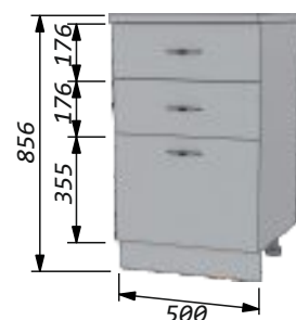
Стол 50 с тремя ящиками.
