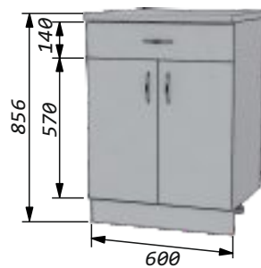
№007 Стол 60 с одним ящиком. Ширина - 600мм Высота - 856мм Глубина: по столешнице - 600мм по корпусу - 460мм
