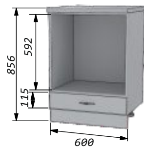
Стол-встройка 60 с ящиком. Ширина - 600мм Высота - 856мм Глубина: по столешнице - 600мм по корпусу - 460мм
