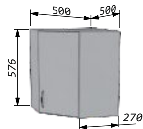
Шкаф угловой скошенный 50х50 глухой правый/левый Ширина - 500х500мм Высота - 576мм Глубина - 270мм
