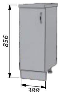
Стол 30 без ящика правый/ левый Ширина - 300мм Высота - 856мм Глубина: по столешнице - 600мм по корпусу - 460мм
