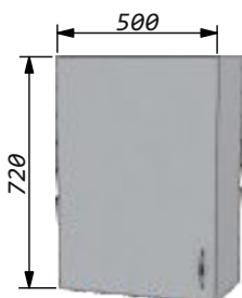
Шкаф глухой 50 правый/левый Ширина - 500мм Высота - 720мм Глубина - 270мм
