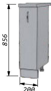
Стол-бутылочница 20 под выдвижную корзину. Ширина -200мм Высота -856мм Глубина: по столешнице-600мм по корпусу -460мм
