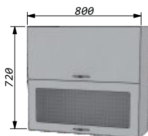
Шкаф-витрина 80 х2 открывание вверх Ширина - 800мм Высота - 720мм Глубина - 270мм
