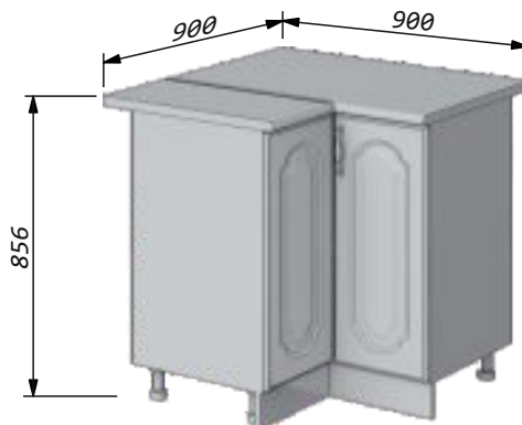
Стол угловой прямой 90x90 правый/левый Размер: по столешнице - 900x900мм по корпусу - 800x800мм Глубина: - по боковому срезу столешницы - 600мм - по боковине корпуса - 460мм Ширина фасада: 313мм и 329мм Длина цоколя: - 716мм
