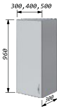
Шкаф глухой 30/40/50 правый/левый Ширина -300/400/500мм Высота -960мм Глубина-300мм
