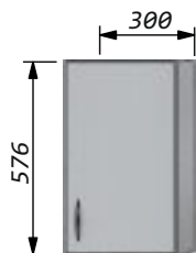
Шкаф-скос 30 малый с фасадом (петли 30 градусов) Ширина -300мм Высота -576мм Глубина-270мм
