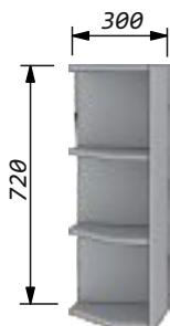
Шкаф-скос 30 граненый Ширина - 300мм Высота - 720мм Глубина - 273мм
