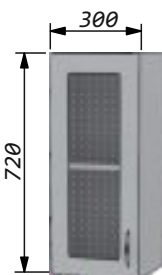
Шкаф-витрина 30 правый/ левый Ширина - 300мм Высота - 720мм Глубина - 270мм
