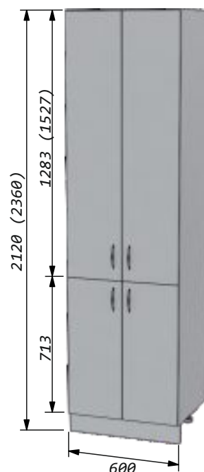
Пенал 60 четыре двери Ширина -600мм Высота -2120мм Глубина-561мм
