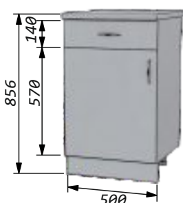
Стол 50 с одним ящиком правый/левый
