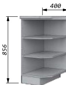
Стол-скос 40 граненый Ширина - 400мм Высота - 856мм Глубина: по столешнице - 600мм по корпусу - 564мм
