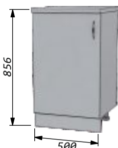
Стол 50 без ящика правый/левый Ширина - 500мм Высота - 856мм Глубина: по столешнице - 600мм по корпусу - 460мм
