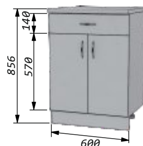
Стол 60 с фальш-ящиком под врезку варочной панели Ширина -600мм Высота -856мм Глубина: по столешнице-600мм по корпусу -460мм
