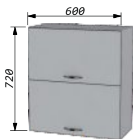
Шкаф 60 х2 глухой открывание вверх Ширина - 600мм Высота - 720мм Глубина - 270мм
