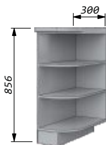
Стол-скос 30 скругленный Ширина - 300мм Высота - 856мм Глубина: по столешнице - 600мм по корпусу - 564мм
