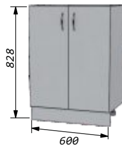
Стол-мойка 60 без ящика Ширина - 600мм Высота - 856мм Глубина по корпусу - 460мм
