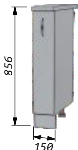
Стол-бутылочница 15 под выдвижную корзину. Ширина -150мм Высота -856мм Глубина: по столешнице-600мм по корпусу -460мм
