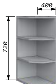
Шкаф-скос 40 граненый Ширина - 400мм Высота - 720мм Глубина - 273мм
