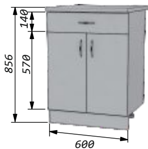
Стол 60 с одним ящиком. Ширина - 600мм Высота - 856мм Глубина: по столешнице - 600мм по корпусу - 460мм
