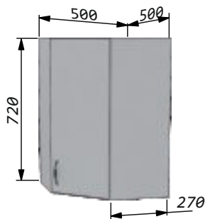
Шкаф угловой 50x50 правый/левый Ширина - 500x500мм Высота - 720мм Глубина - 270мм
