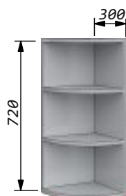
Шкаф-скос 30 скругленный Ширина - 300мм Высота - 720мм Глубина - 273мм
