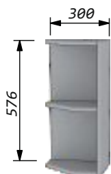
Шкаф-скос 30 малый граненый Ширина - 300мм Высота - 576мм Глубина - 273мм
