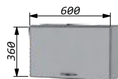
Шкаф-под вытяжку 60 открывается вверх.
