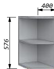
Шкаф-скос 40 малый скругленный Ширина - 400мм Высота - 576мм Глубина - 273мм
