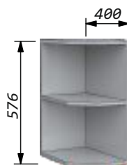
Шкаф-скос 40 малый граненый Ширина - 400мм Высота - 576мм Глубина - 273мм
