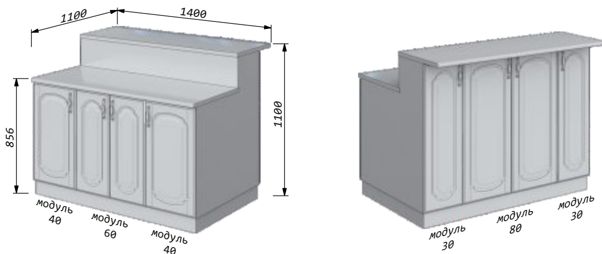
Кухонный остров тип 2 - барный
