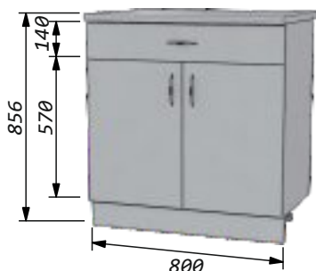
Стол 80 с одним ящиком Ширина - 800мм Высота - 856мм Глубина: по столешнице - 600мм по корпусу - 460мм
