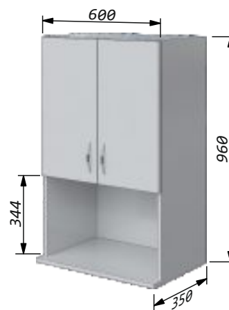
Шкаф 60 под микроволновку Ширина - 600мм Высота - 960мм Глубина по боковинам - 300мм
