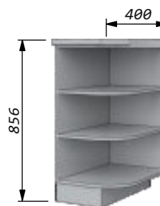
Стол-скос 40 скругленный Ширина - 400мм Высота - 856мм Глубина: по столешнице - 600мм по корпусу - 564мм
