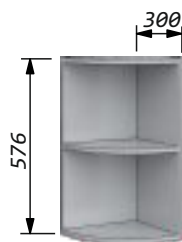
Шкаф-скос 30 малый скругленный Ширина - 300мм Высота - 576мм Глубина - 273мм
