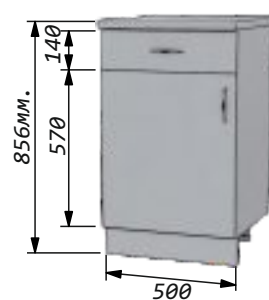
Стол 50 с одним ящиком правый/левый Ширина - 500мм Высота - 856мм Глубина: по столешнице - 600мм по корпусу - 460мм
