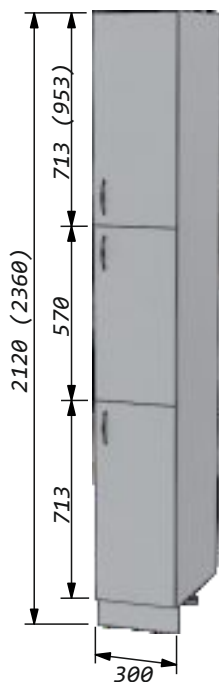
Пенал 30 три двери правый/левый Ширина -400мм Высота -2120мм Глубина-561мм
