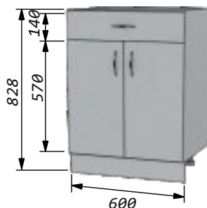
Стол-мойка 60 с фальш-ящиком. Ширина - 600мм Высота - 856мм Глубина по корпусу - 460мм
