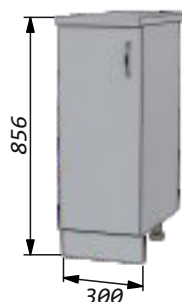
Стол 30 без ящика правый/левый Ширина - 300мм Высота - 856мм Глубина: по столешнице - 600мм по корпусу - 460мм
