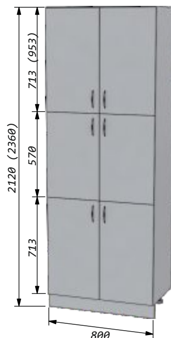
Пенал 80 шесть дверей Ширина - 800мм Высота - 2120мм Глубина - 561мм
