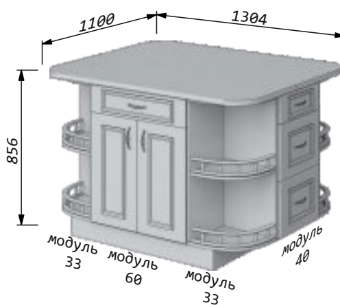
Кухонный остров тип 7 (одноуровневый скруглённый с баллюстрадами)
