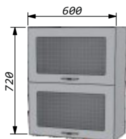
Шкаф-витрина 60 х2 с 2 стеклами открывание вверх Ширина - 600мм Высота - 720мм Глубина - 270мм
