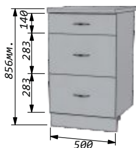
№00 Стол 50 с тремя ящиками. Ширина - 500мм Высота - 856мм Глубина: по столешнице - 600мм по корпусу - 460мм
