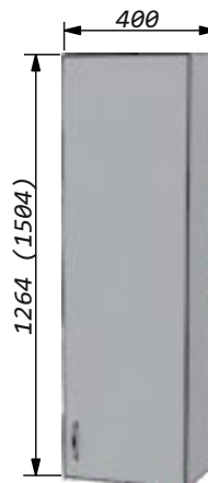
Пенал 40 настольный правый/левый Ширина - 400мм Высота - 1264мм Глубина - 270мм
