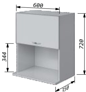
Шкаф 60 под микроволновку Ширина - 600мм Высота - 720мм Глубина по боковинам - 270мм
