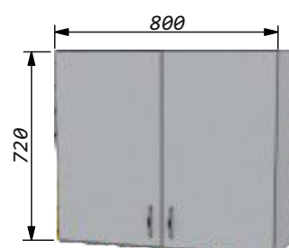
Шкаф глухой 80 Ширина - 800мм Высота - 720мм Глубина - 270мм
