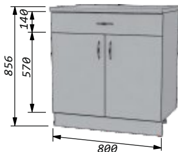
№001 Стол 80 с одним ящиком Ширина - 800мм Высота - 856мм Глубина: по столешнице - 600мм по корпусу - 460мм
