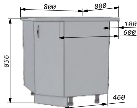
Стол угловой скошенный 80x80, правый правый/левый Размер: по столешнице - 800x800мм по корпусу - 700x700мм Глубина: - по срезу столешницы - 600мм - по боковине корпуса - 460мм Ширина фасада: - 310мм Длина цоколя - 355мм
