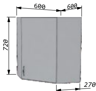
Шкаф угловой 60х60 правый/левый
