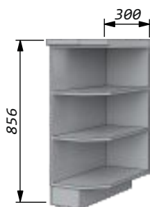
Стол-скос 30 граненый Ширина - 300мм Высота - 856мм Глубина: по столешнице - 600мм по корпусу - 564мм
