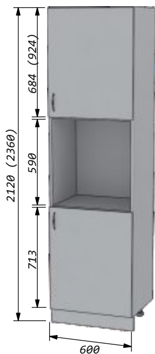
Пенал-встройка 60 правый/левый Ширина - 400мм Высота - 2120мм Глубина - 561мм
