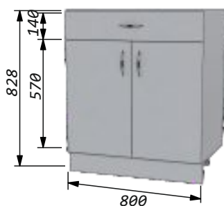
Стол-мойка 80 с фальш-ящиком. Ширина -800мм Высота -856мм Глубина по корпусу -460мм
