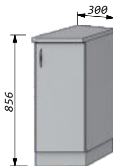
Шкаф-скос 30 с фасадом (петли 30 градусов) Ширина -300мм Высота -856мм Глубина: по столешнице-600мм по корпусу -561мм Применяется в сочетании с «шкафом-скосом 30 с фасадом»
