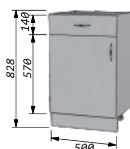
Стол-мойка 50 с фальш-ящиком правый/левый
