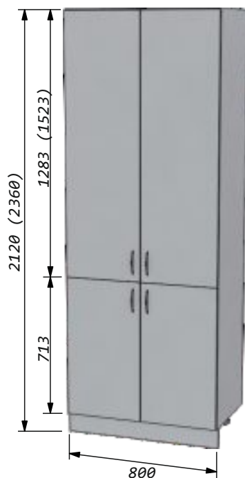
Пенал 80 четыре двери Ширина - 800мм Высота - 2120мм Глубина - 561мм
