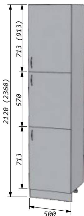
Пенал 50 три двери правый/левый Ширина -400мм Высота -2120мм Глубина-561мм
