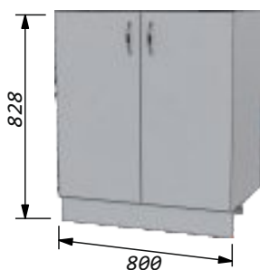
Стол-мойка 80 без ящика Ширина -800мм Высота -856мм Глубина по корпусу -460мм
